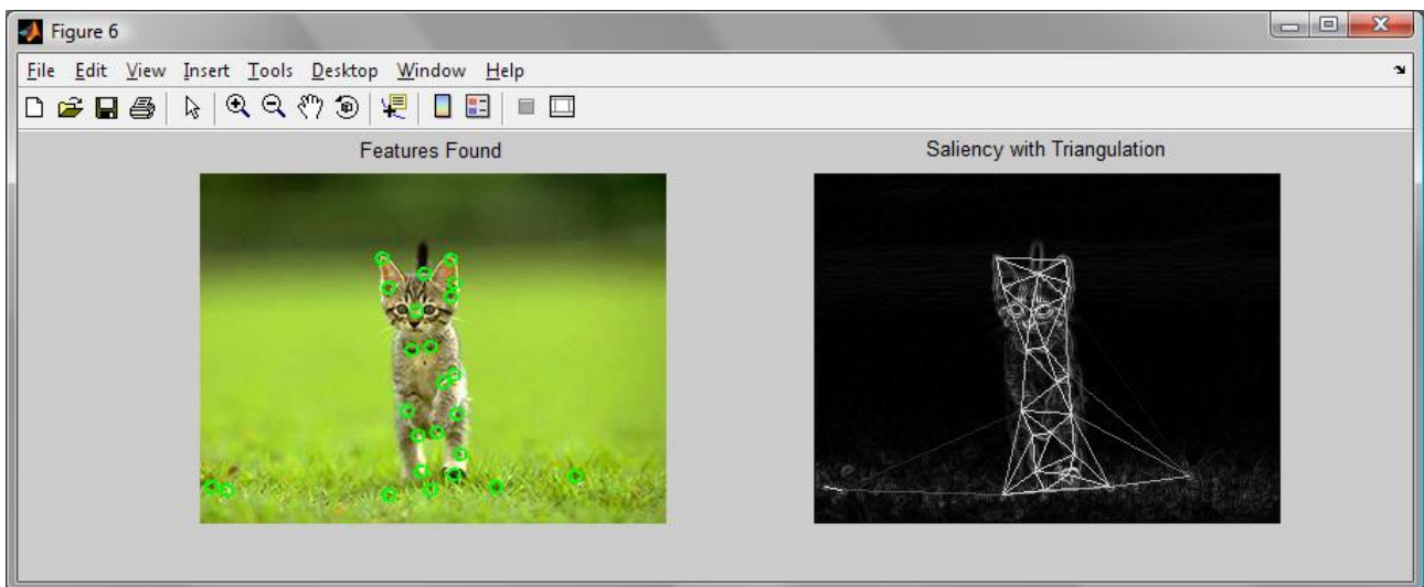
FIGURA 5 Quest'esempio mostra il risultato ottenuto dalla ricerca delle features e come queste siano utilizzate per modificare la funzione energia. Nell'immagine a sinistra è stato utilizzato l'Harris Corner Detection individuando le features che sono state evidenziate da dei cerchietti verdi. Nell'immagine a destra viene mostrata la funzione energia. Il nero determina il valore 0 mentre il bianco il massimo valore presente. Utilizzando le features è stata disegnata la griglia di Delaunay facendo attenzione ad usare intensità diverse per segmenti di lunghezza diversa. Più questi sono lunghi, più si confonderanno col nero dello sfondo, indicando una minore importanza.
