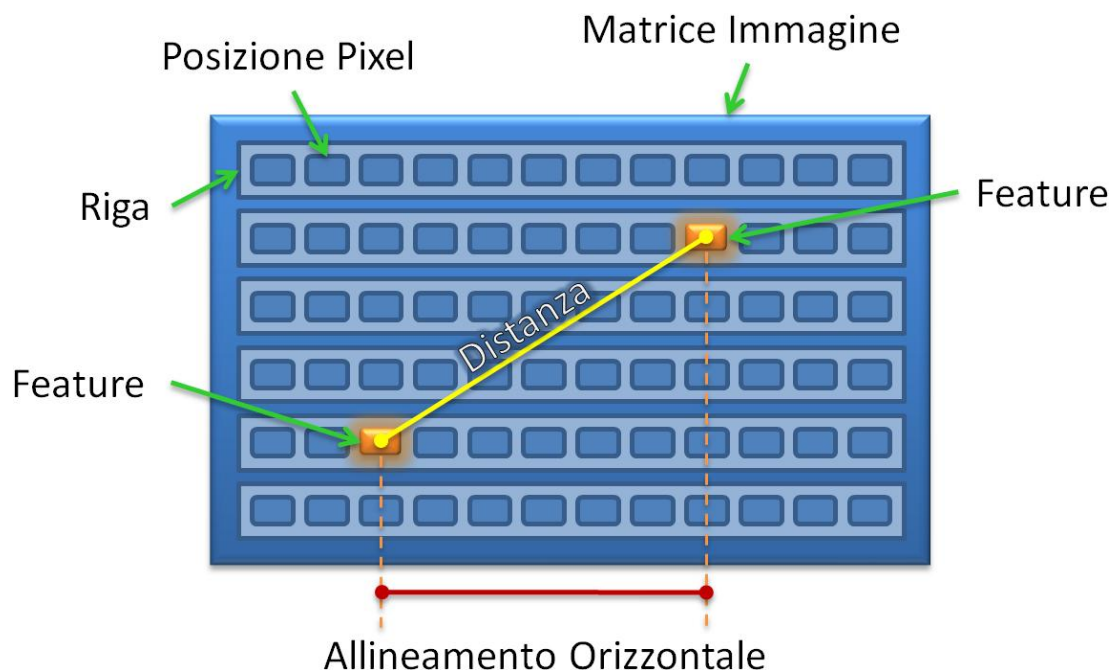
FIGURA 6 Lo schema mostra la struttura dell'immagine. Come è evidenziato, ogni riga è considerata indipendentemente dalle altre. I vincoli definiti rispetto alle features impongono l'allineamento orizzontale tra i pixel interessati, mentre il peso del vincolo è inversamente proporzionale alla loro distanza.
